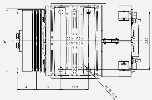
Det. Z-Z
